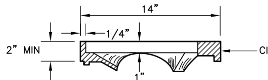
RISER RING
